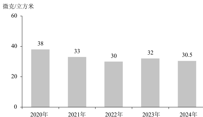
图 9 2020-2024 年细颗粒物 (PM 2.5 ) 年均浓度
